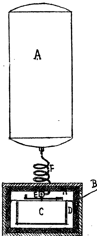
Appareil Cailletet pour la prise d'air dans les hautes régions atmosphériques.
